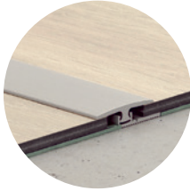
Perfil de dilatación de vinyl NEVREXPSILV 2.000 × 32,5 × 7,5 mm
